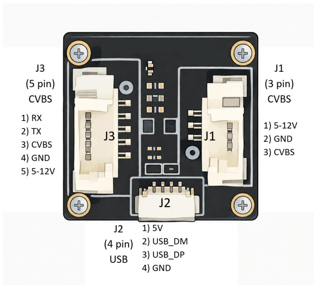
Fig.2. Diagrama de cableado
