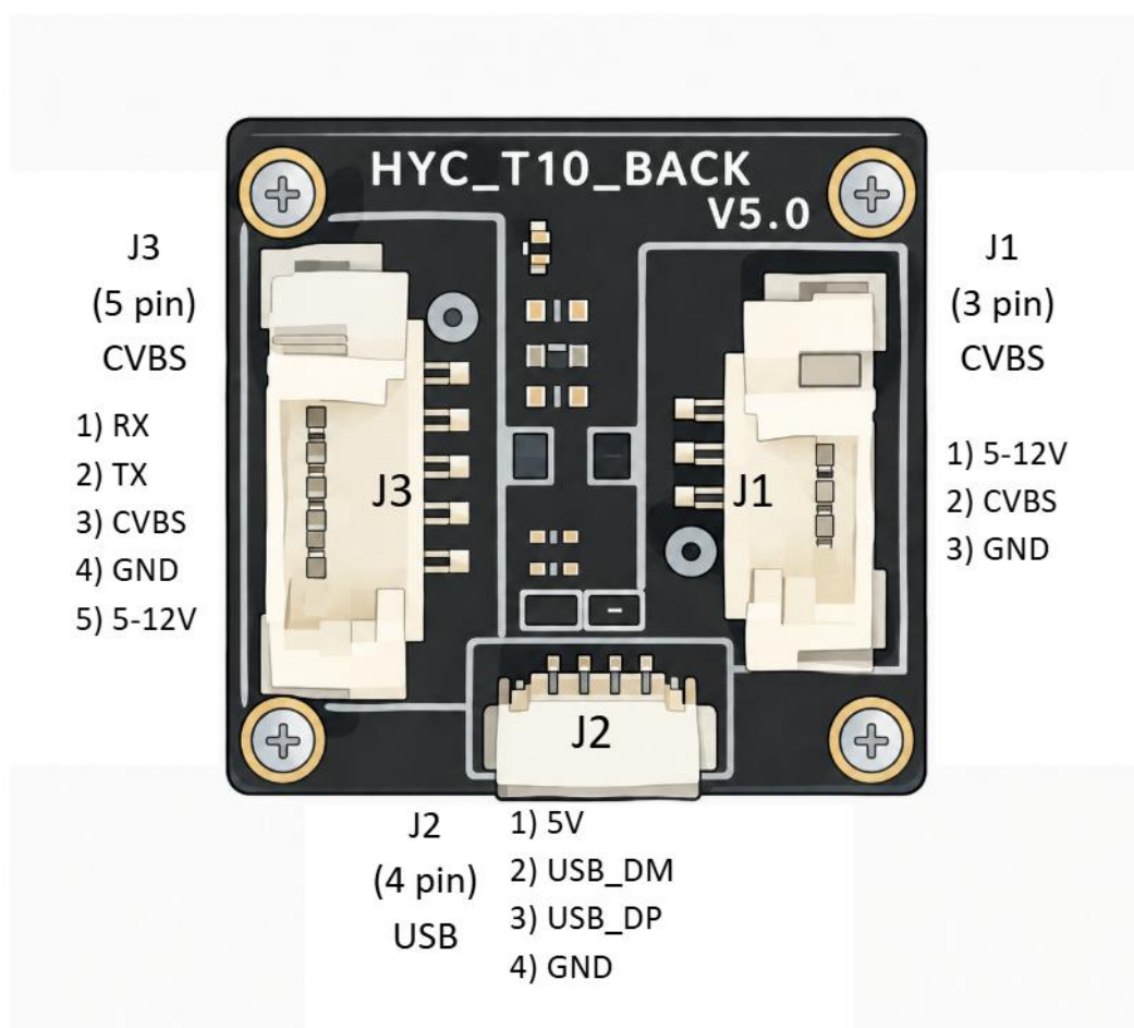
Rys.2. Schemat okablowania
