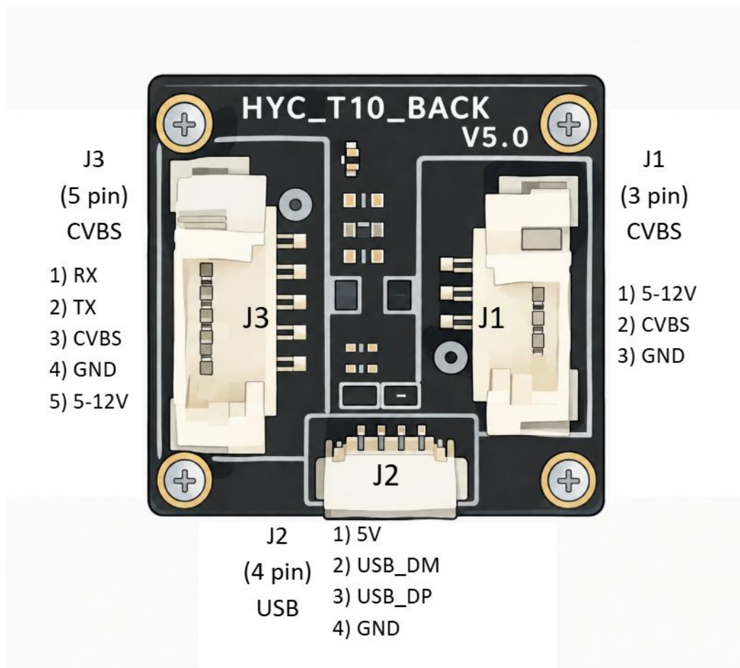
Fig.2. Schema di cablaggio
