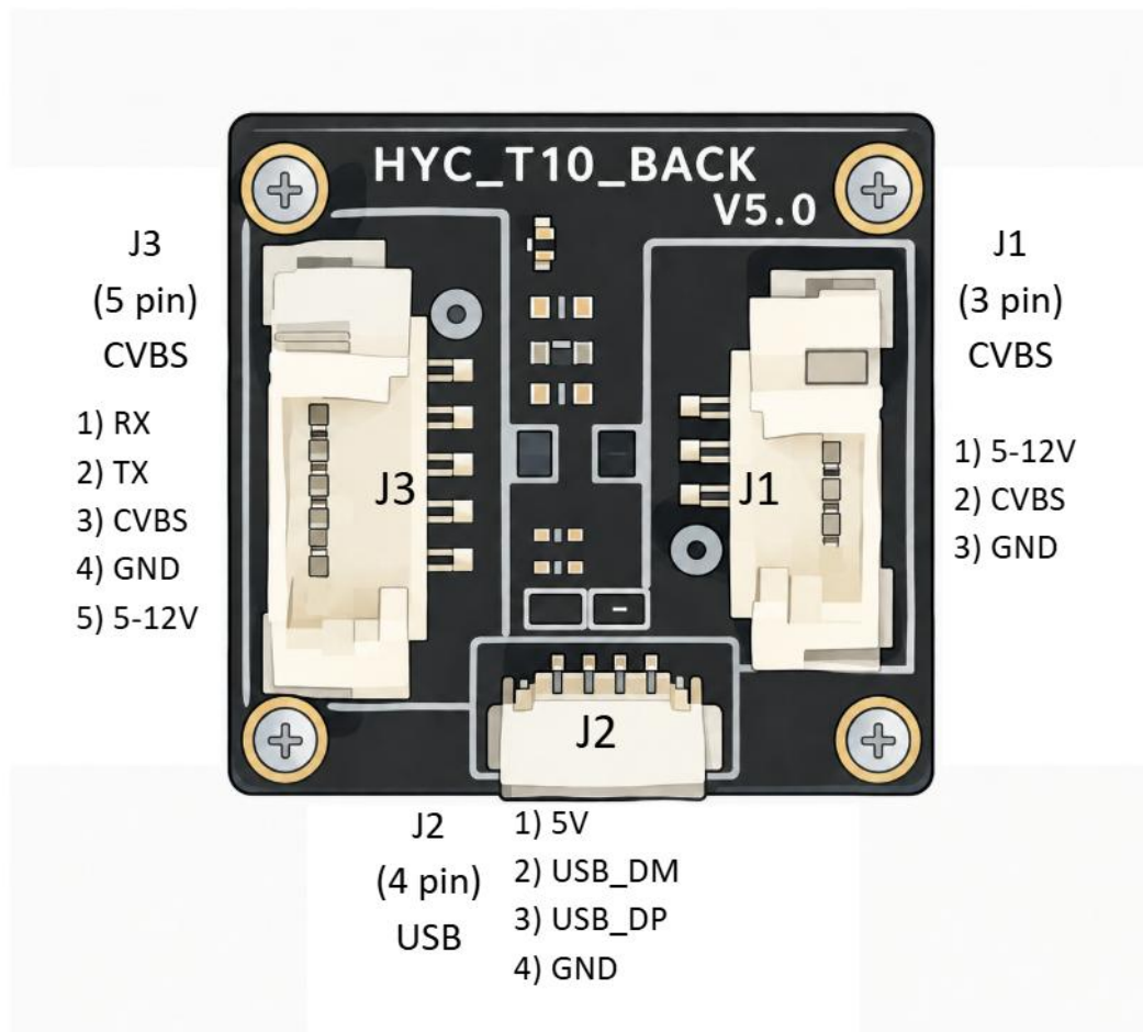
Abb.2. Verkabelungsschema
