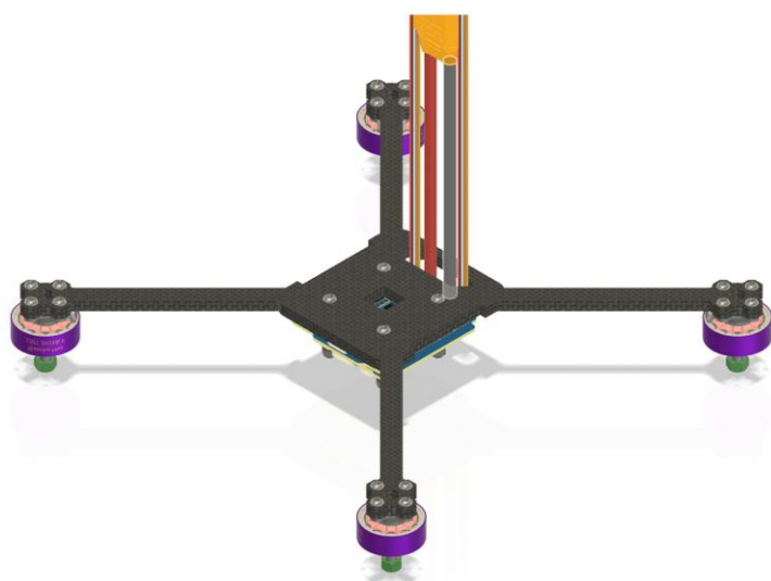
Рис. 4. Збірка двигунів
