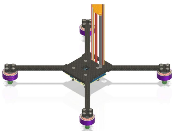
Obr. 4. Montáž motorů
