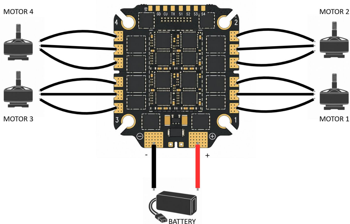
Мал.2. Схема розведення дротів
