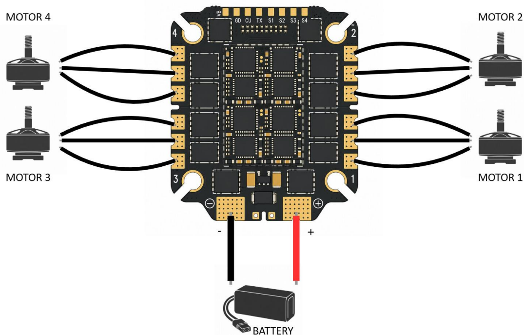
Obr.2. Schéma zapojení
