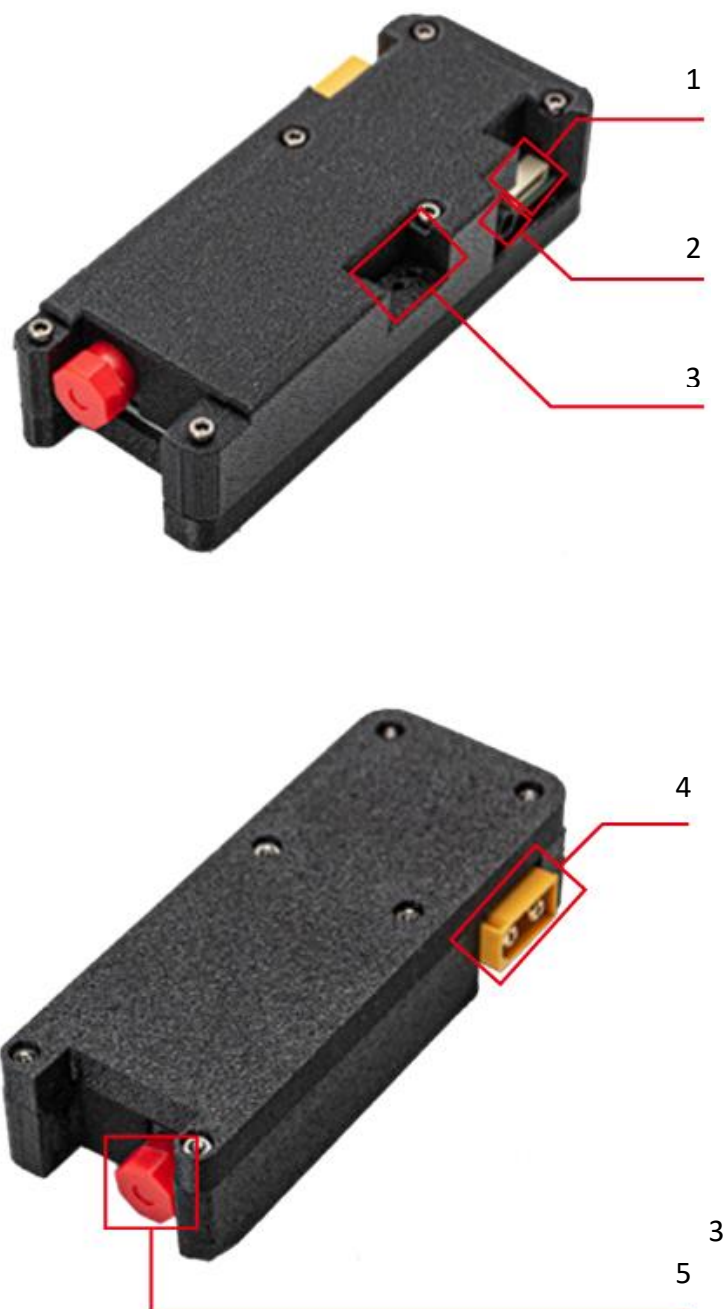
Abb.1. Bodenmodul
