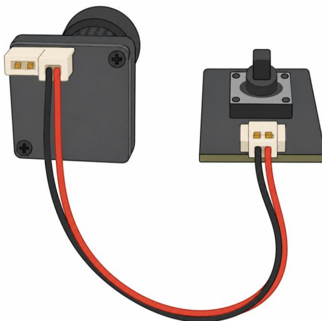
Obr.2. Připojení OSD joysticku
